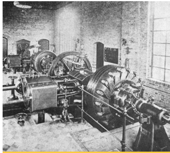
Diese Generatoren lieferten den ersten Strom in Dresden. Zunächst nur für den Betrieb der Straßenbahn, später auch für die erste elektrische Stadtbeleuchtung.
